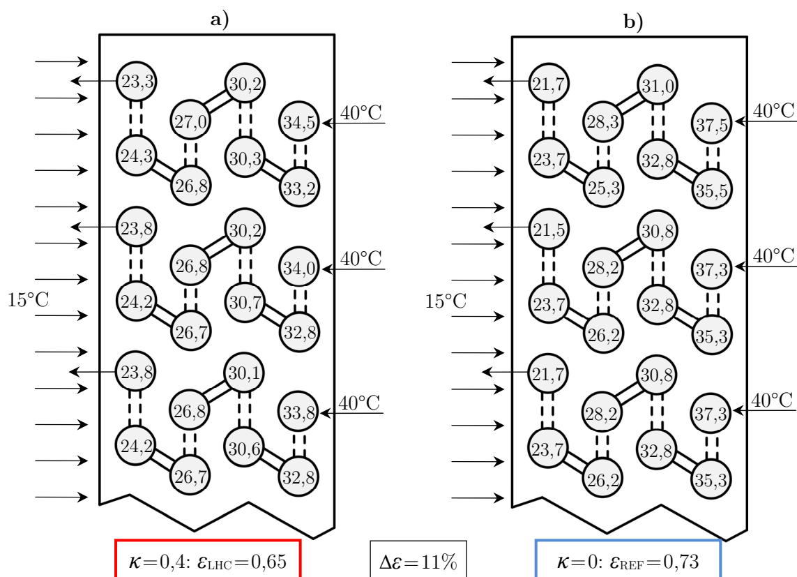
Slika 6.98. Temperature fluida u cijevima izmjenjivača 4R:10×8 ( \pi_2=3 i \pi_3=1 ): a) provođenjem topline u lamelama ( \kappa=0,4 ) i b) bez provođenja topline u lamelama ( \kappa=0 )
