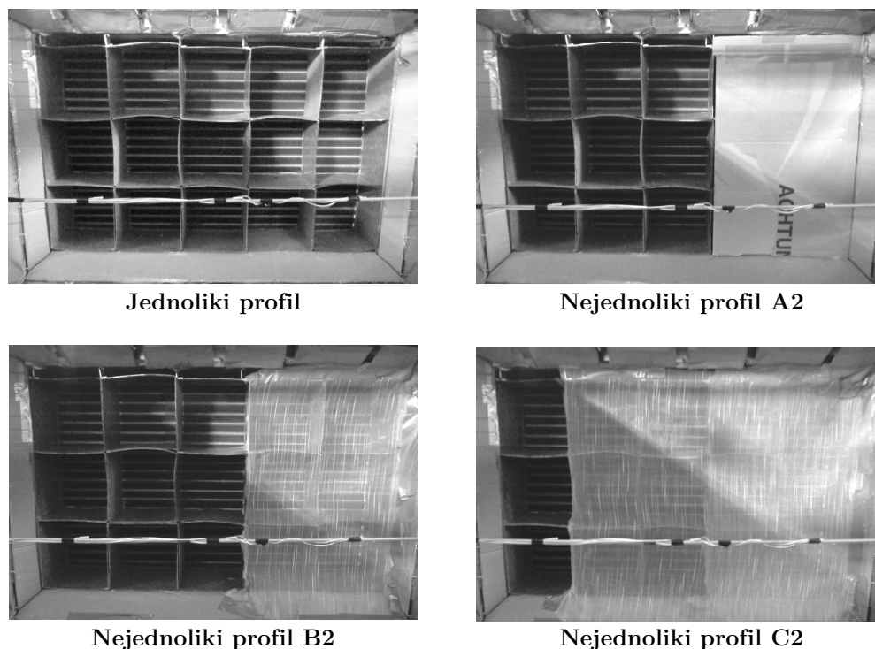
Slika 6.70. Rešetka u zračnom kanalu za dobivanje nejednolikih profila brzina strujanja zraka na ulazu u cijevni lamelni izmjenjivač topline 4R:10×8
