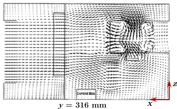
Slika 2.7. Brzina strujanja zraka u kompaktnom klima uređaju dobivena numeričkim modeliranjem (EHA5, Airedale International) [97]
