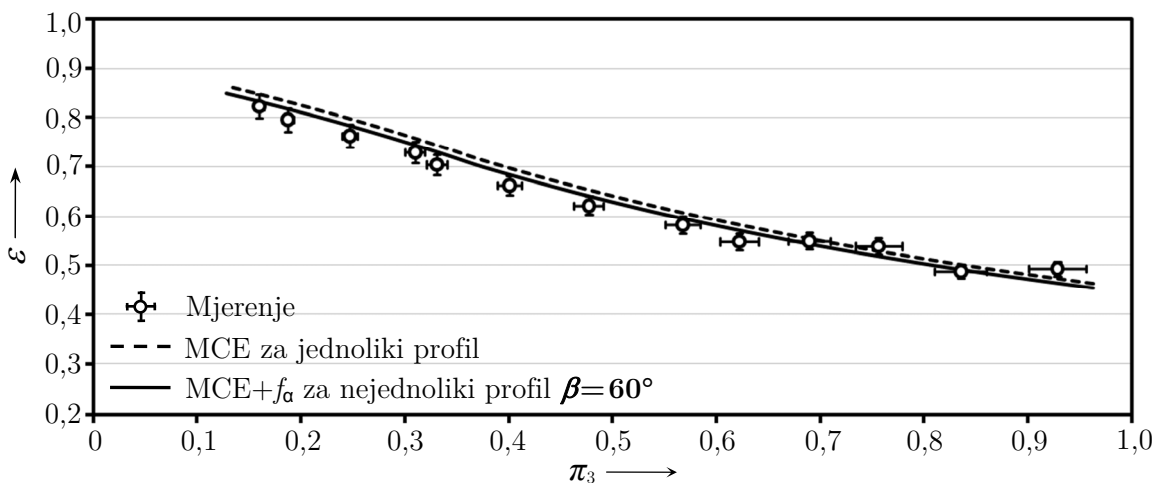
Slika 6.87. Usporedba između rješenja MCE metode i mjerenja iskoristivosti topline u izmjenjivačima 3R:10×6/V:60°
