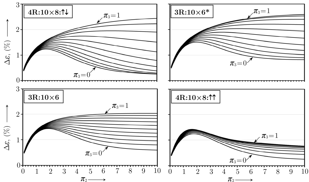
Slika 6.93. Smanjenje iskoristivosti topline u cijevnim lamelnim izmjenjivačima uzrokovano nejednolikim profilom brzina zraka P4 (uz \zeta=0,33 i B=0,55 )
