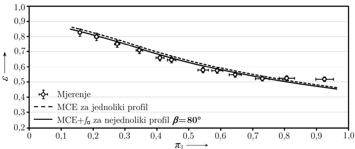
Slika 6.88. Usporedba između rješenja MCE metode i mjerenja iskoristivosti topline u izmjenjivačima 3R:10×6/V:80°
