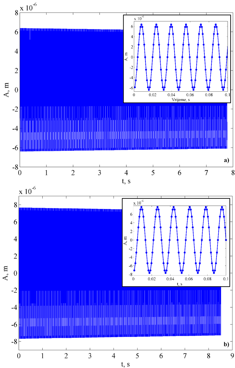
Slika 66. Profil uzbude uklještenja pri ubrzanju od 1 \text{ m/s}^2 za frekventijski raspon od: a) 63 do 64,5 Hz i b) 57,5 do 59 Hz
