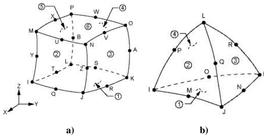
Slika 53. a) Prizmatični SOLID186 i b) tetraedarski SOLID187 3D konačni elementi [Ansys Inc. 2 , 1994.]
