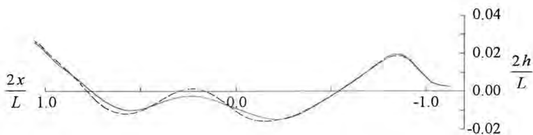
Sl. 8.25. Profil vala forme K5 (—) i osnovne forme (---)
