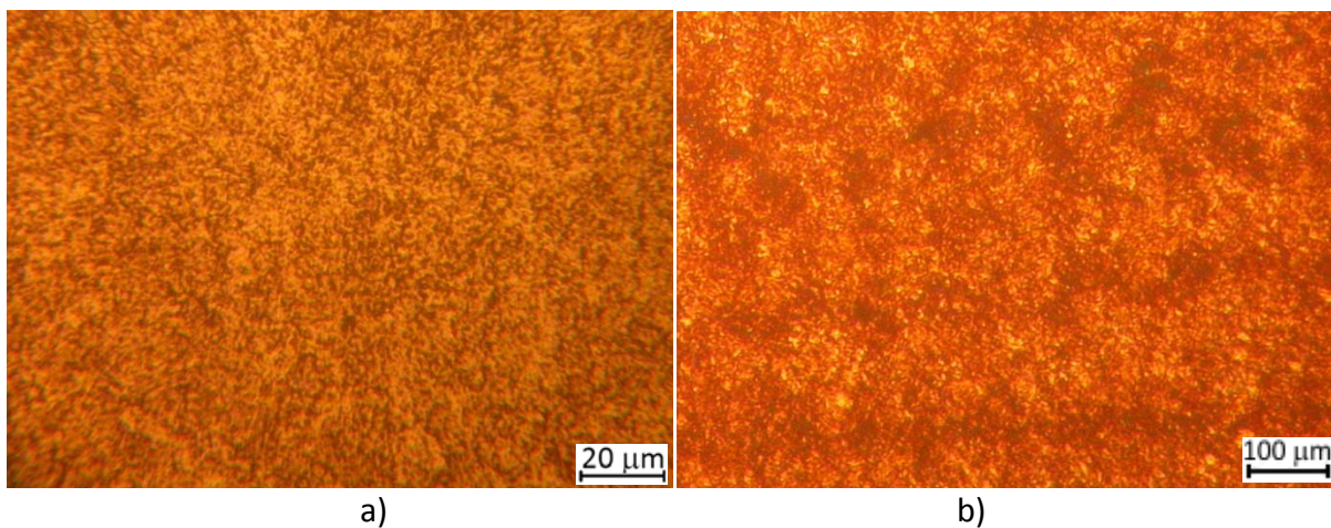
Slika 4.25. Metallografski snimak uzorka 1 nakon poboljšavanja, a) nagrizano 2 %-tnom \text{HNO}_3 u alkoholu, 500:1, b) nagrizano pikrinsko-solnom kiselinom, 100:1
