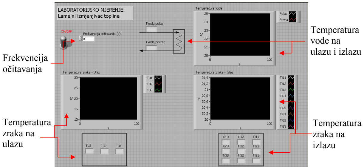
Sl. 4.19. Virtualni instrument razvijen u LabView -u
