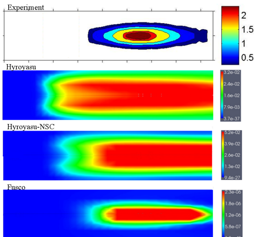
Slika 4.1.45: Usporedba koncentracije čađe dobivena različitim modelima s eksperimentalno izmjerenom koncentracijom
