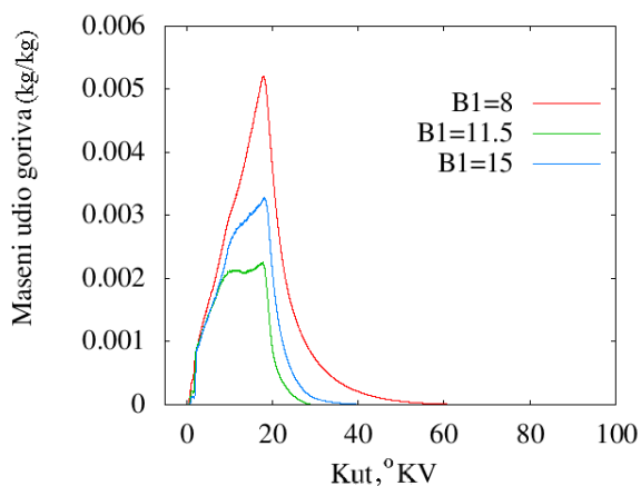
Slika 5.17: Utjecaj koeficijenta B1 na maseni udio goriva u cilindru
