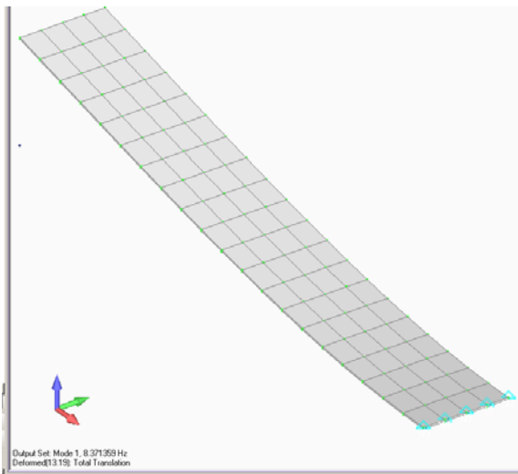
Slika 4.11. Provjera frekvencije 1. oblika vibriranja
