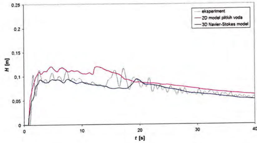
Slika 4.28. Proračunate razine vode na mjernom mjestu G3
