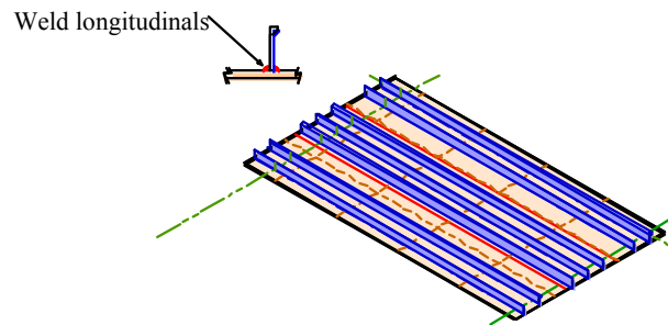
Fig. 3.59. Longitudinal welding [2]
