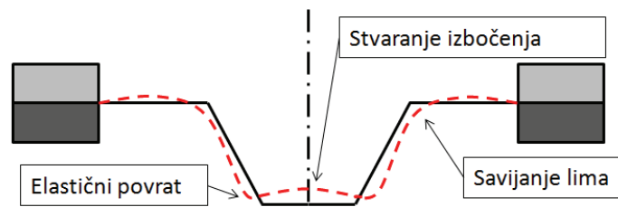
Slika 2.25 Odstupanje konačne geometrije od zadanog oblika [59]
