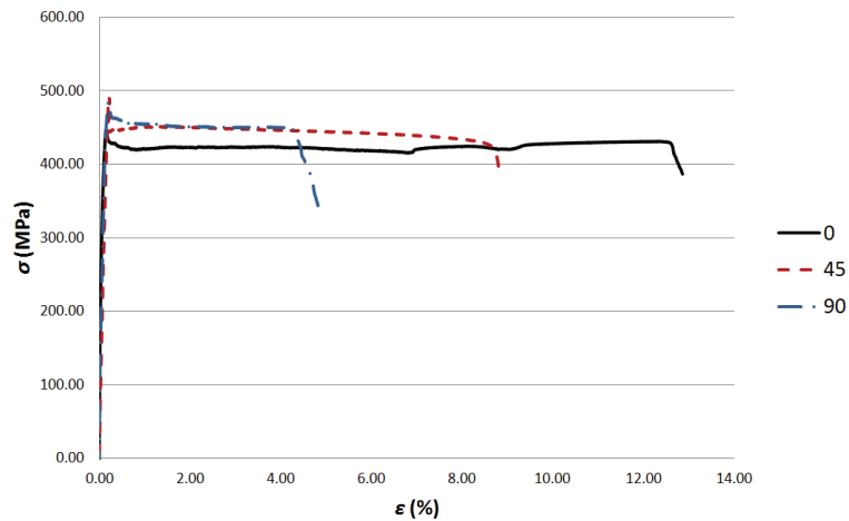
Slika 5.6 Dijagram \sigma - \varepsilon - materijal TH415, kut 0^\circ , 45^\circ , 90^\circ , žarene epruvete A_{80}
