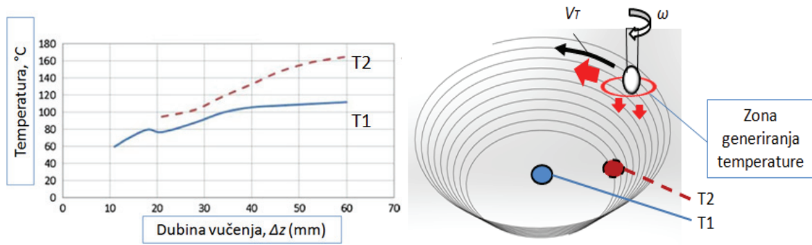
Slika 2.20 Temperatura krnjeg stošca mjerena termoparima T1 i T2 za materijal AA6082 - T6, kut 52,5° [49]
