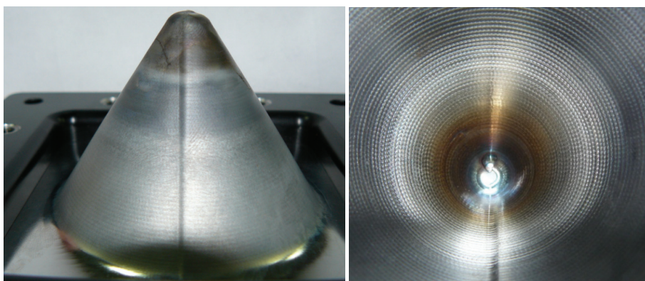
Slika 8.14 Prikaz izratka TH415 (uzorak x1) izvučenog sa konstantnom brzinom i bez podmazivanja, pregrijavanje lima na visini od 35 mm gdje se temperatura kreće iznad 180^\circ\text{C} , kut od 57^\circ
