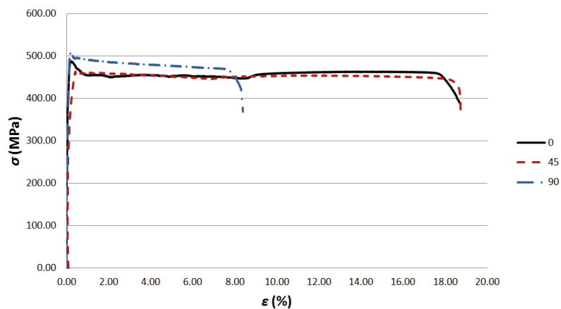
Slika 5.7 Dijagram \sigma - \varepsilon - materijal TH415, kut 0^\circ , 45^\circ , 90^\circ , žarene epruvete A_{40}
