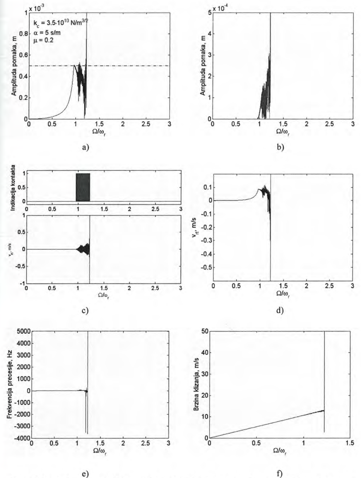
Slika 4.21. a) Odziv rotora pri ubrzanju kroz kritičnu brzinu sa realnim parametrima nelinearnog modela kontakta te koeficijentom trenja \mu=0.2 , b) Odziv statora, c) Relativna normalna brzina između rotora i statora sa indikacijom kontakta, d) Tangencijalna brzina središta diska rotora, e) Frekvencija precesije rotora, f) Brzina klizanja u dodirnoj točki rotora i statora
