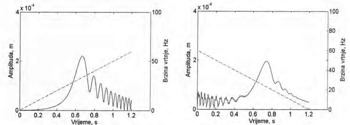
Slika 4.1. Tranzijentni odziv rotora pri kutnom ubrzanju \varepsilon = 100\pi , \text{rad/s}^2 (odnosno usporenju \varepsilon = -100\pi , \text{rad/s}^2 )
