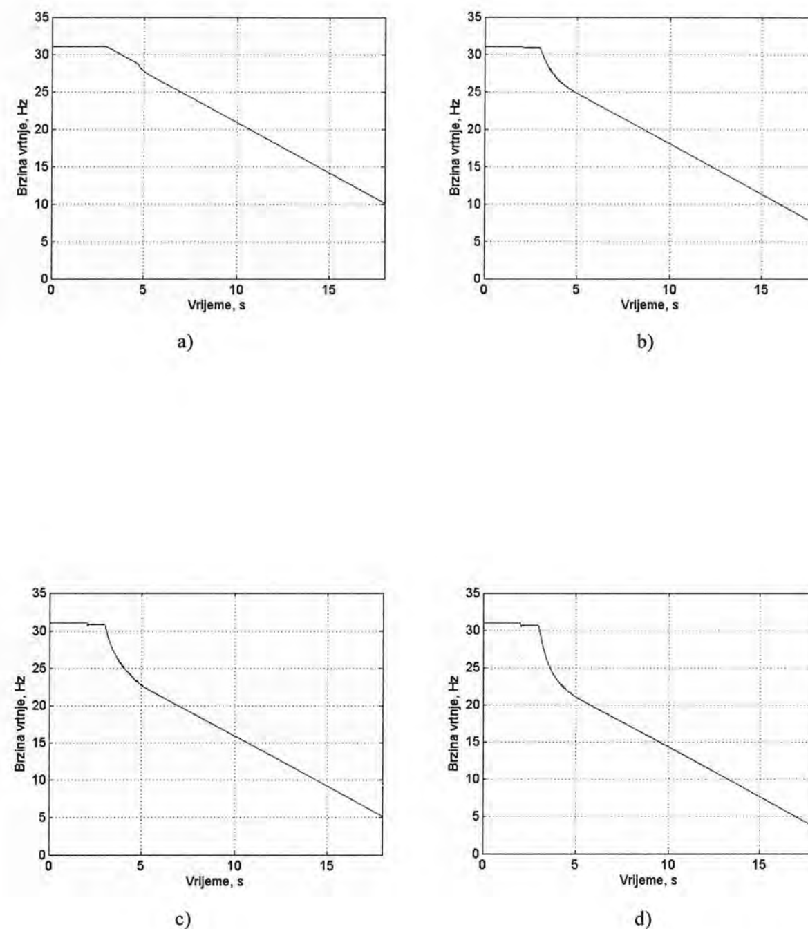
Slika 4.52. Brzina vrtnje rotora za slijedeće mase otpadnute lopatice: a) m_{add} = 1 \cdot 10^{-3} kg, b) m_{add} = 5 \cdot 10^{-3} kg, c) m_{add} = 11 \cdot 10^{-3} kg, d) m_{add} = 20 \cdot 10^{-3} kg,
