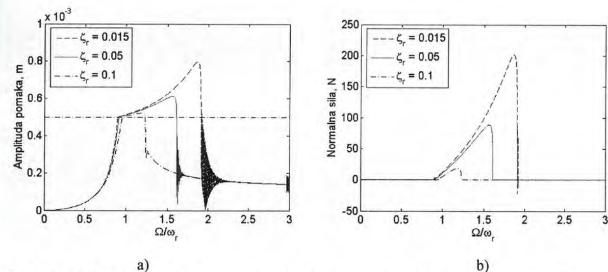
Slika 4.15. Odzivi rotora pri ubrzanju kroz kritičnu brzinu pri različitim omjerima prigušenja rotora \zeta_r , a) Amplitude pomaka, b) Normalne sile dodira F_N
