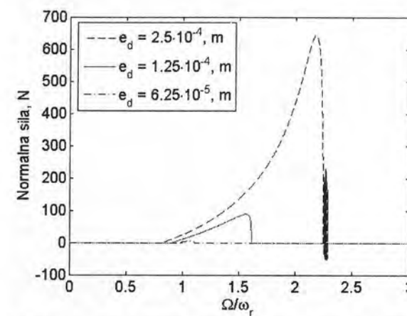
Slika 4.14. Odzivi rotora pri ubrzanju kroz kritičnu brzinu pri različitim iznosima neuravnoteženja, c) Normalne sile dodira pri različitim neuravnoteženjima
