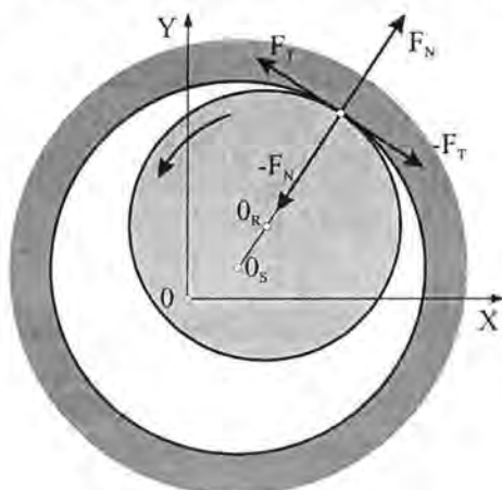
Slika 2.8. Definicija sile u kontaktu koje djeluju na rotor odnosno stator
