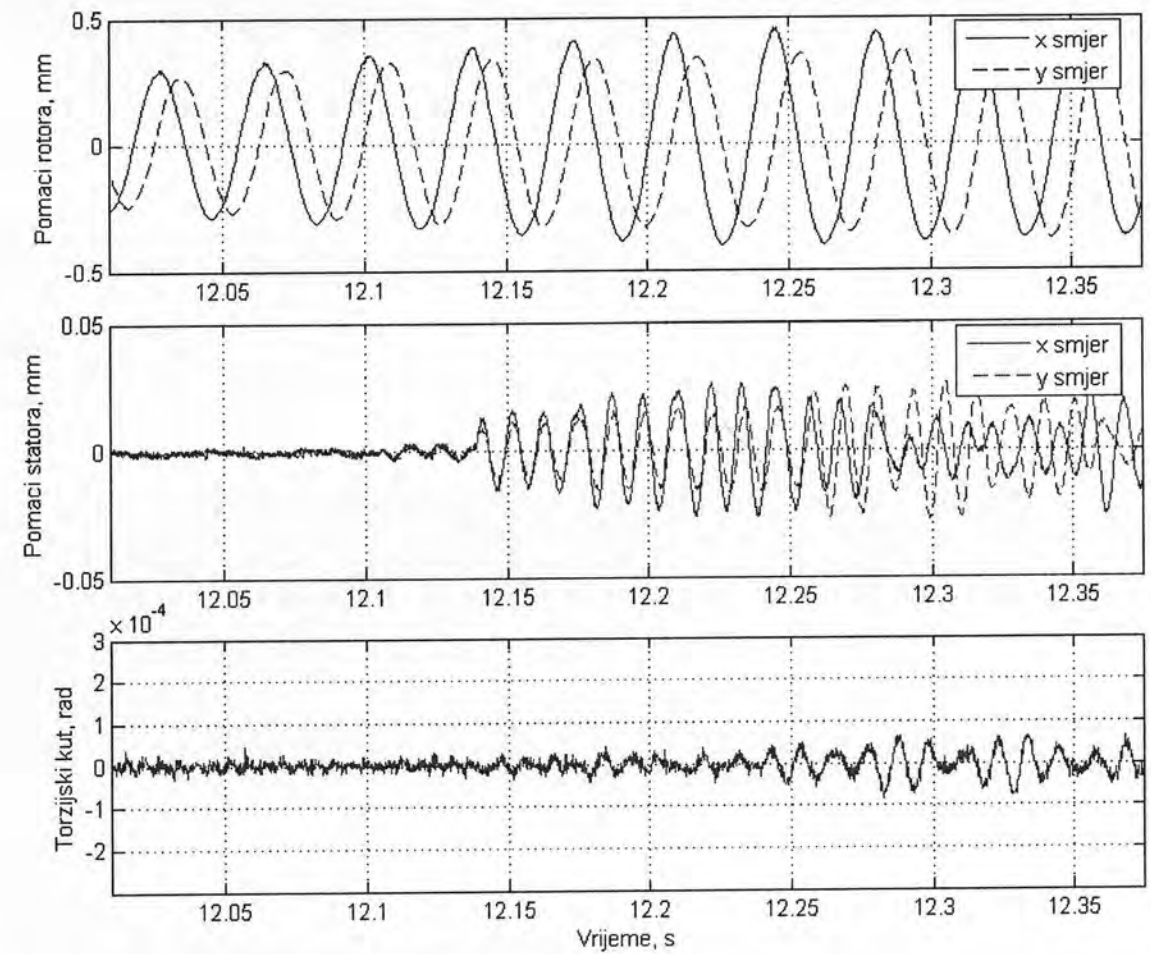
Slika 6.23. Poprečni pomaci rotora i statora te torzijski kut statora u vremenskoj domeni pri brzini vrtnje n = 27.21 Hz
