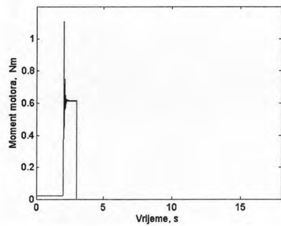
Slika 4.57. Moment motora, simulacija d) m_{add} = 20 \cdot 10^{-3} kg
