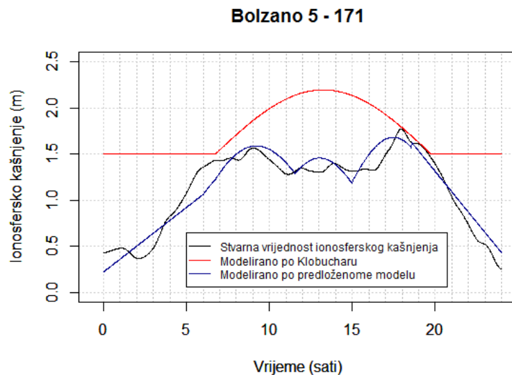
Slika 6.6: Stvarno ionosfersko kašnjenje, ionosfersko kašnjenje modelirano prema Klobucharu te prema predloženoj modelu na stanici Bolzano (Italija) za dan 171 u 2006. godini
