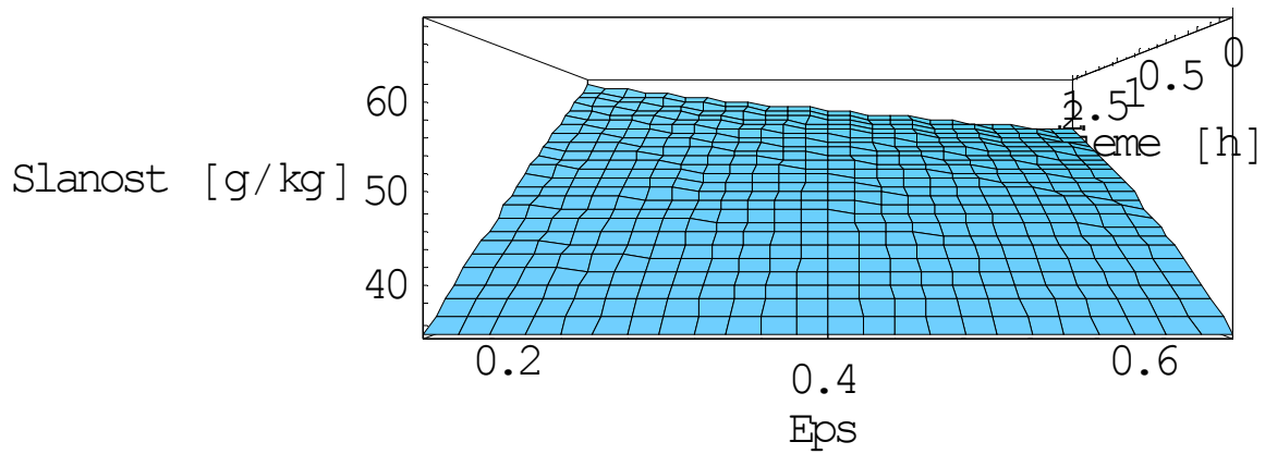
Slika 4.24. Trodimenzionalni prikaz izraza 4.3.2 za D/M_o\varepsilon=0,5
