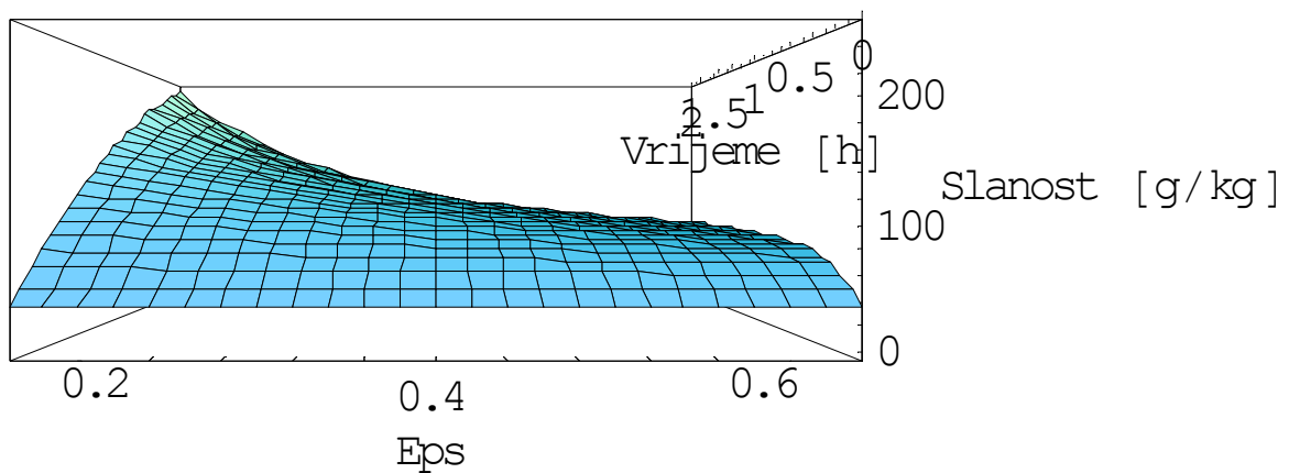
Slika 4.29. Trodimenzionalni prikaz izraza 4.3.2 za D/M_o\varepsilon=5
