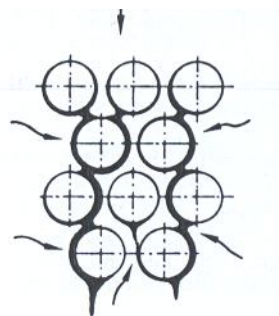
Slika 3.11. Kondenzacija na snopu cijevi
