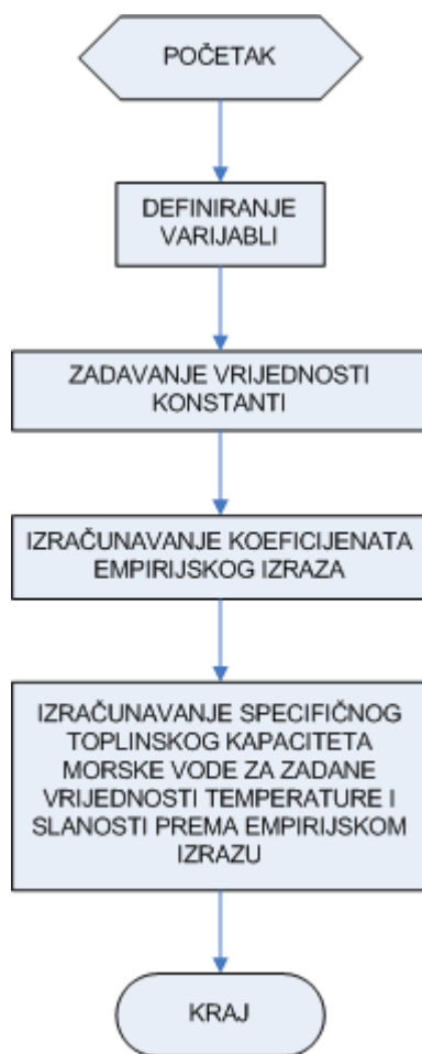
Slika 4.5. Blok dijagram potprograma za određivanje specifičnog toplinskog kapaciteta morske vode
