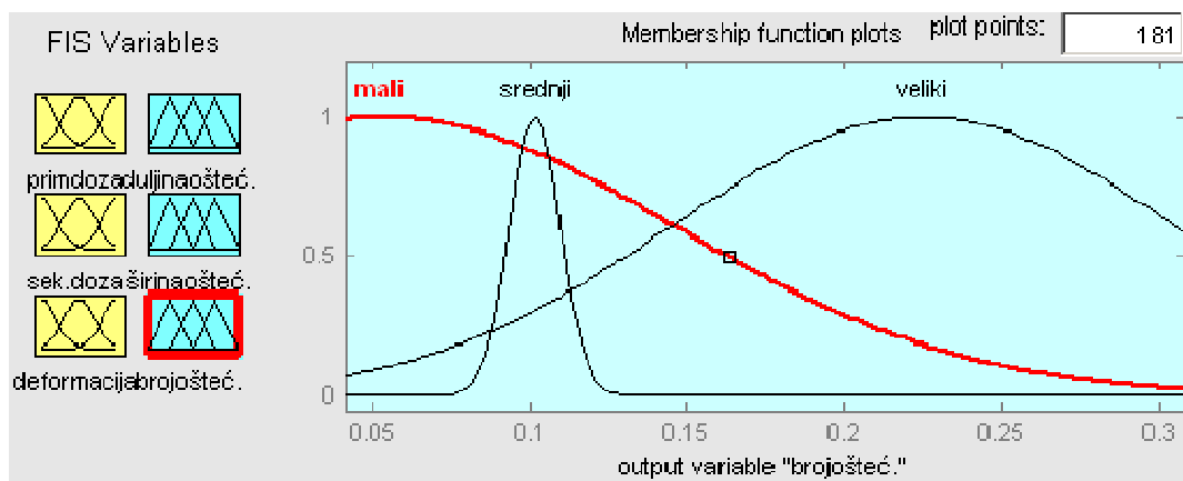
Slika 51. Oblici funkcija pripadnosti izlazne varijable broj oštećenja
