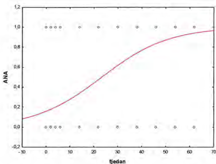
Slika 19: Predviđanje nalaza ANA modelom logističke regresije. Na ordinatnoj osi vrijednost 0 označava ANA negativni, a vrijednost 1 pozitívni nalaz. Točke predstavljaju prikupljene podatke ANA nalaza u grupi ispitanika.
