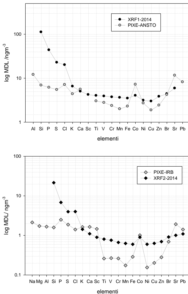
Slika 6.3. Usporedba prosječnih donjih granica detekcije elemenata (MDL) u \text{ngm}^{-3} na različitom skupu uzoraka. Gore: PIXE-ANSTO i XRF1-2014 analiza aerosola uzorkovanih 2012. godine; Dolje: PIXE-IRB i XRF2-2014 analiza aerosola uzorkovanih 2013. i 2014. godine
