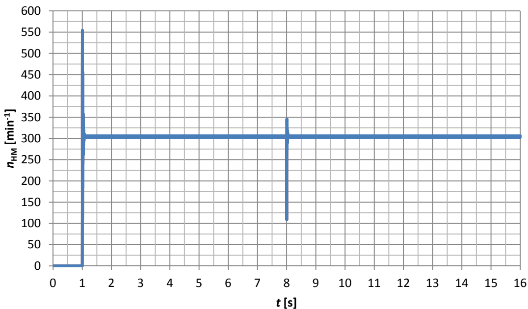
Slika 6.8. Brzina vrtnje hidromotora kod prvog testa modela
