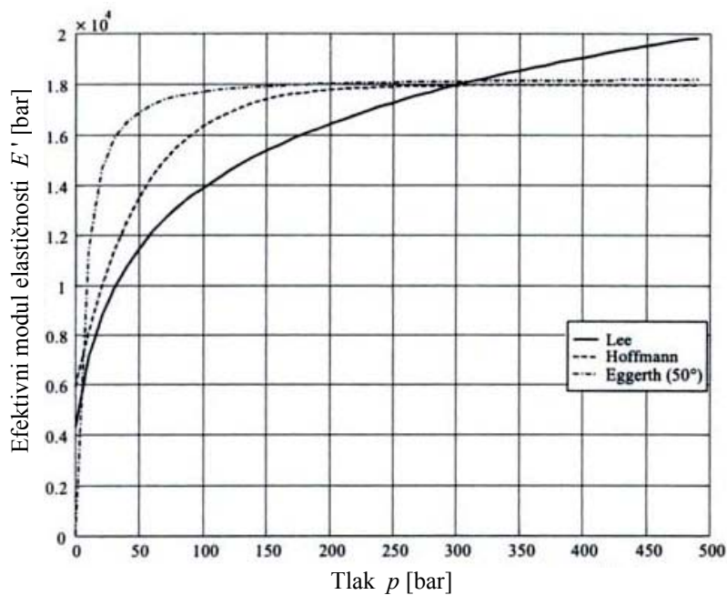
Slika 3.2. Usporedba različitih jednačnji za izračunavanje E' [65]
