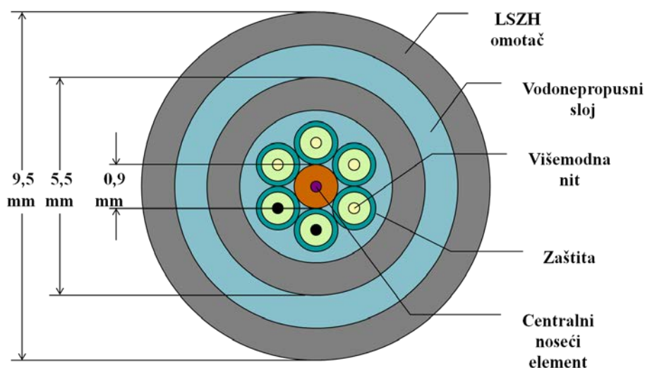
Slika 61: Presjek svjetlovnog LSZH kabela s 4 višemodne niti
