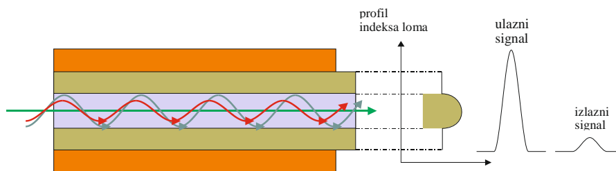
Slika 29: Rasprostiranje svjetlosti kroz višemosnu nit s gradijentnim profilom indeksa loma
