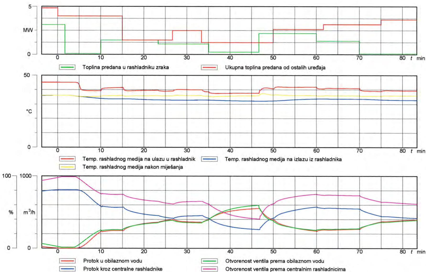
Sl. 6.19 Simulacija proizvoljnoga toplinskog opterećenja rashladnog sistema (NT krug rashlade, morska voda 32 ^{\circ}\text{C} )
