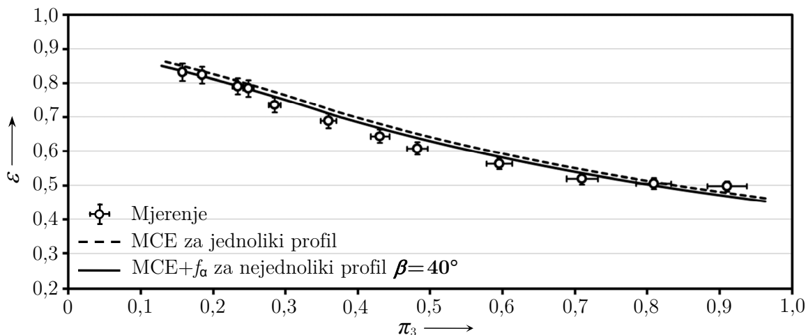
Slika 6.86. Usporedba između rješenja MCE metode i mjerenja iskoristivosti topline u izmjenjivačima 3R:10×6/V:40°
