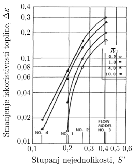
Slika 1.3. Smanjenje iskoristivosti topline u unakrsnom pločastom izmjenjivaču topline u ovisnosti o stupnju nejedolikosti profila ulaznih brzina strujanja fluida [7]
