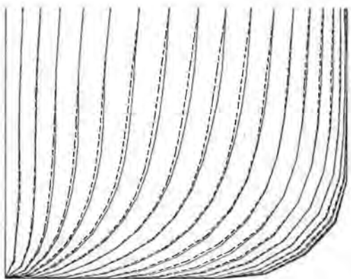
Sl. 8.11. Pramčana rebra forme P5 (—) i osnovne forme (---)
