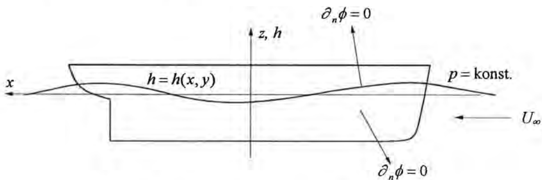
Sl. 2.2. Rubni uvjeti za potencijalno strujanje
