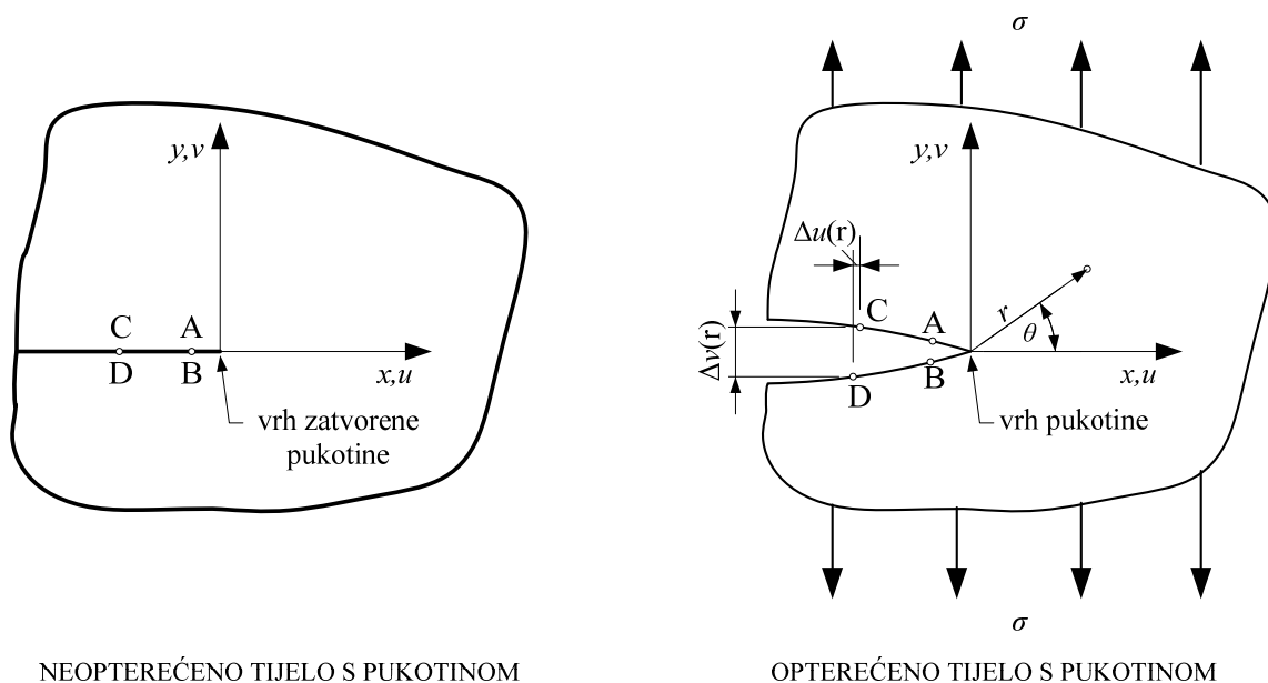
Slika 5.3 Relativni pomaci površina pri otvaranju pukotine
