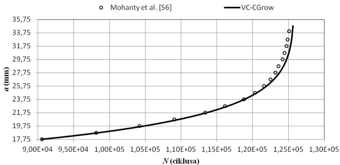
Slika 7.23 Rast pukotine u zavisnosti od broja ciklusa za primjer 1
