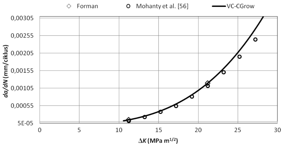
Slika 7.30 Zavisnost prirasta pukotine od raspona faktora intenziteta naprezanja za primjer 2
