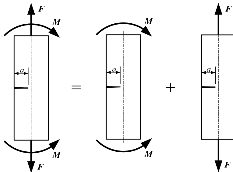
Slika 3.8 Kombinirano opterećenje elementa koji sadrži pukotinu
