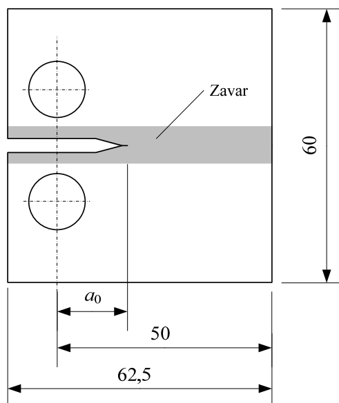
Slika 7.16 Dimenzije C(T) epruvete korištene za primjer 4 [77]
