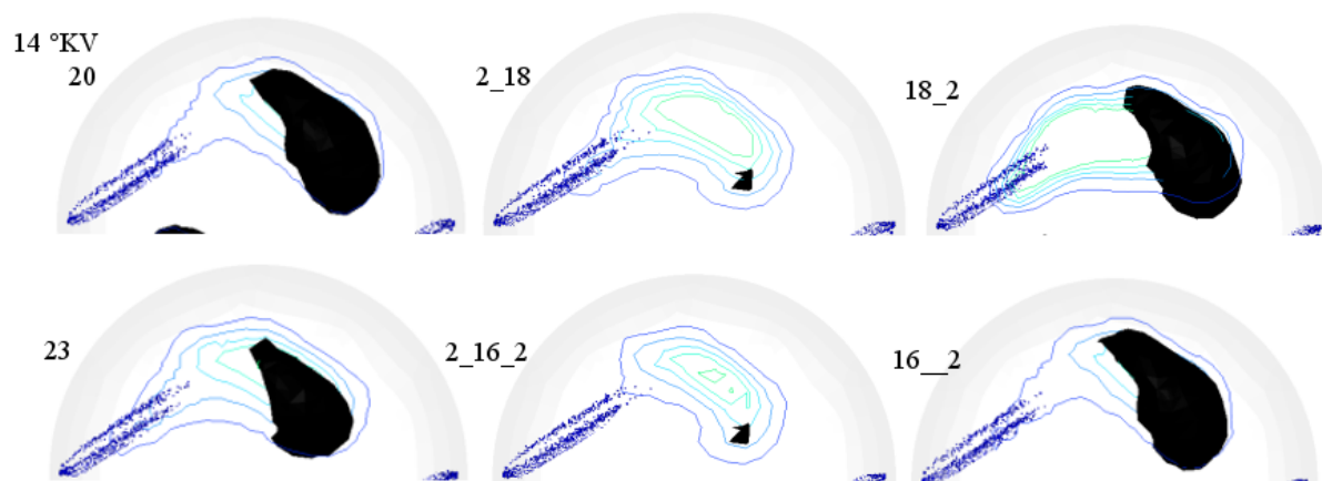
Slika 5.52: Kapljice goriva, isolinije masenih udjela pare goriva od 0.01, 0.03, 0.05, 0.07 i 0.09 kg/kg, isoploha volumnog udjela čađe od 0.0005 cm 3 /cm 3 za trenutak 14 °KV
