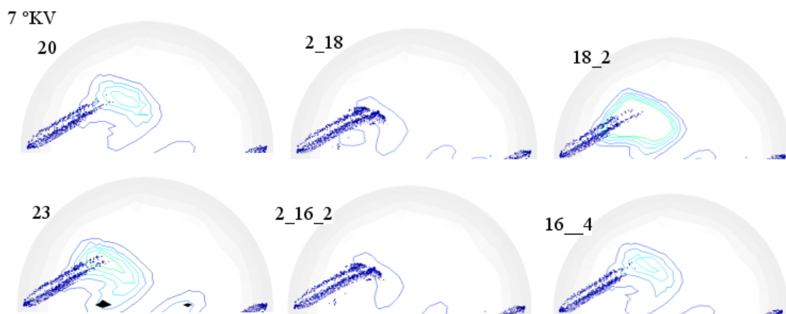
Slika 5.51: Kapljice goriva, isolinije masenih udjela pare goriva od 0.01, 0.03, 0.05, 0.07 i 0.09 kg/kg, isoploha volumnog udjela čađe od 0.0005 cm 3 /cm 3 za trenutak 7 °KV
