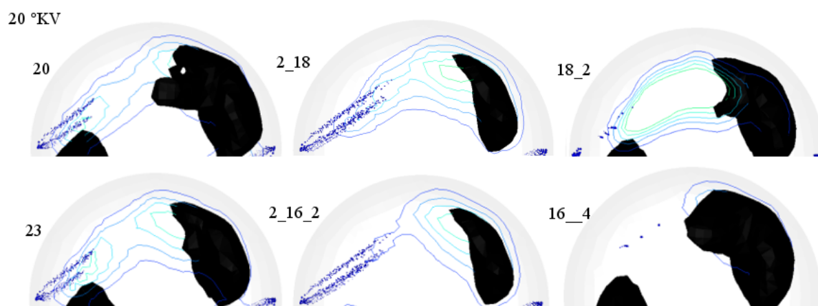
Slika 5.53: Kapljice goriva, isolinije masenih udjela pare goriva od 0.01, 0.03, 0.05, 0.07 i 0.09 kg/kg, isoploha volumnog udjela čađe od 0.0005 cm 3 /cm 3 za trenutak 20 °KV
