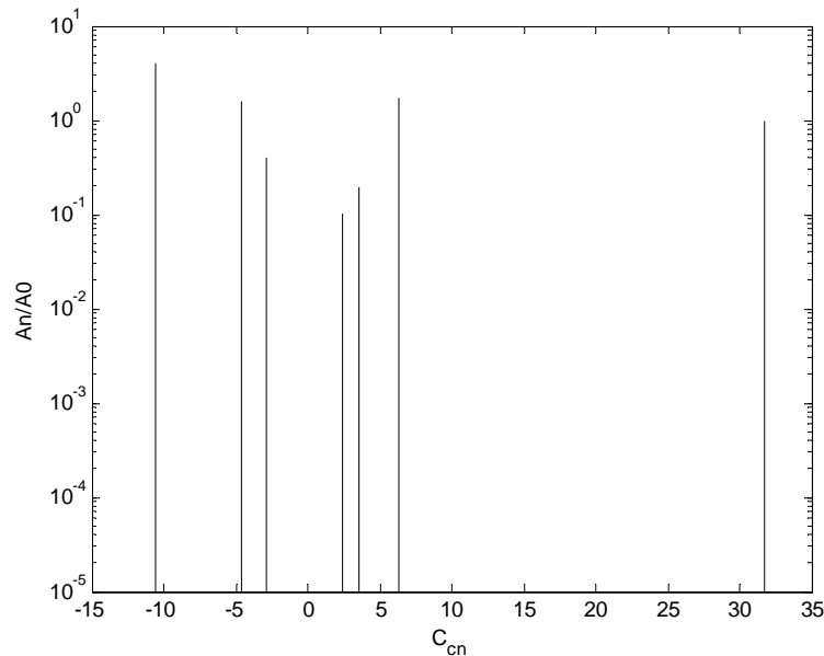
Slika 2.20. Omjer amplituda prostornih harmonijskih valova slobodne valne grupe ( \Omega=50,2 )
