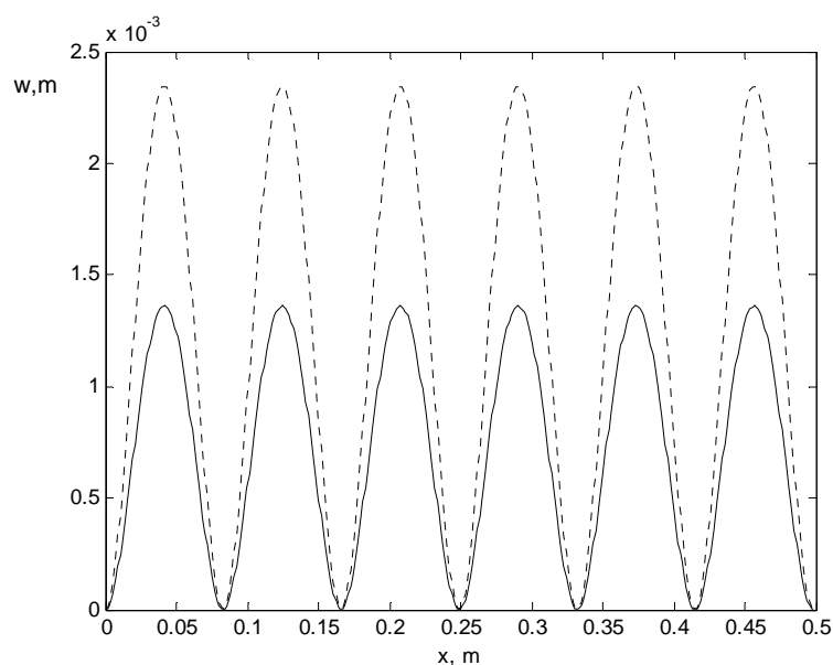
Slika 4.13. Oblik vibriranja na gornjoj graničnoj frekvenciji prvog propagacijskog pojasa izračunat pomoću računalnog modela u Matlab-u, _____ realni i - - - - - imaginarni dio
