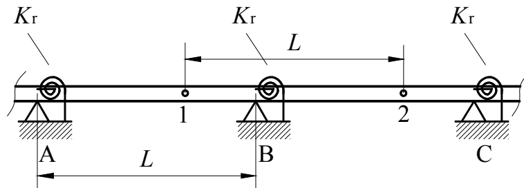
Slika 2.2. Beskonačna greda periodički oslonjena na jednostavne oslonce
