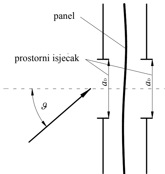
Slika 2.30. Shematski prikaz metode prostornog isječka
