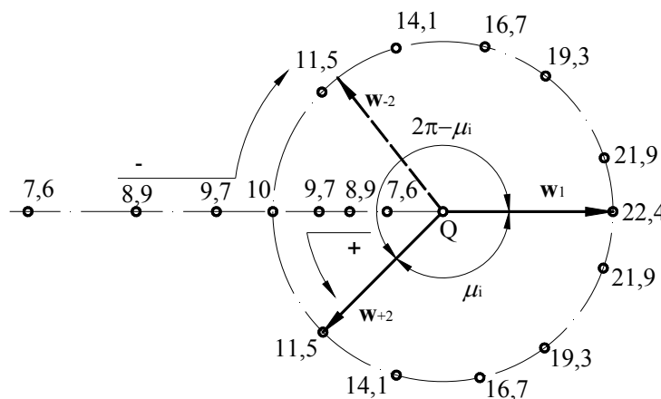
Slika 2.13. Prikaz vektora pomaka w_1 i w_2 u susjednim periodima grede
