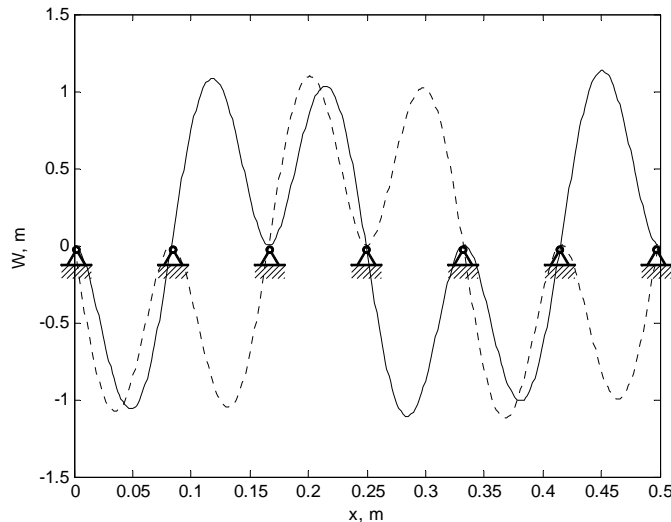
Slika 2.18. Oblik vibriranja pri \Omega=15.5 : realna _____ i imaginarna -----
