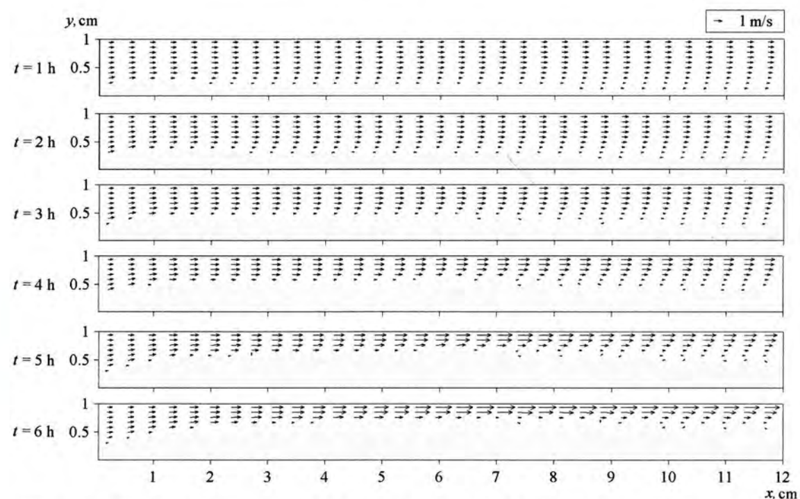
Slika 7.8. Polja vektora brzina strujanja zraka pri ispitivanju I u različitim vremenima dobivena numeričkim putem
