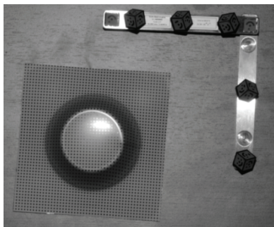
Slika 9.16 Uzorak krnjeg stošca TH415 sa kutom 63^\circ , visina 25 mm, mjereno sustavom ARGUS
