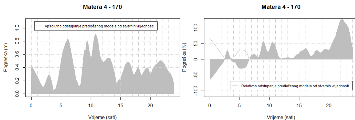
Slika 6.22: Apsolutno (lijevo) i relativno (desno) odstupanje predloženeog modela od stvarnih vrijednosti ionosferskog kašnjenja tijekom 170. dana u 2006. godini – stanica Matera (Italija)
