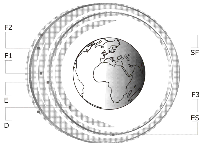
Slika 2.14: Prikaz ionosferskih slojeva u odnosu na međusobni položaj Sunca i Zemlje
