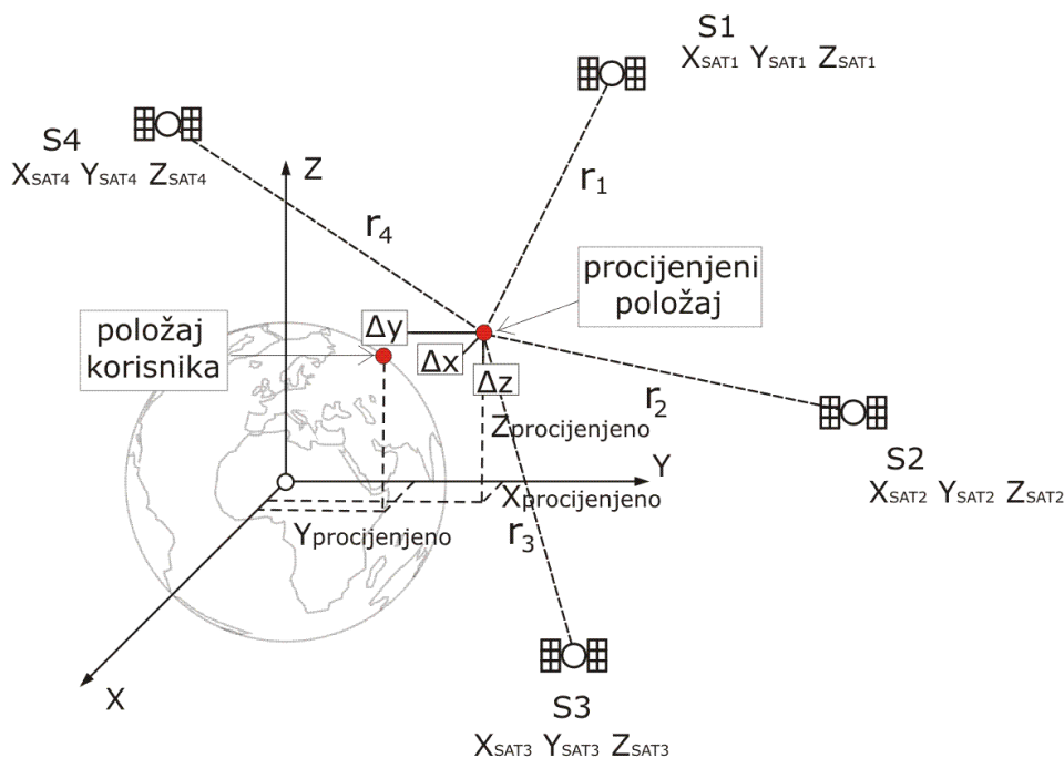
Slika 2.10: Postupak procjene položaja satelitskim navigacijskim sustavima
