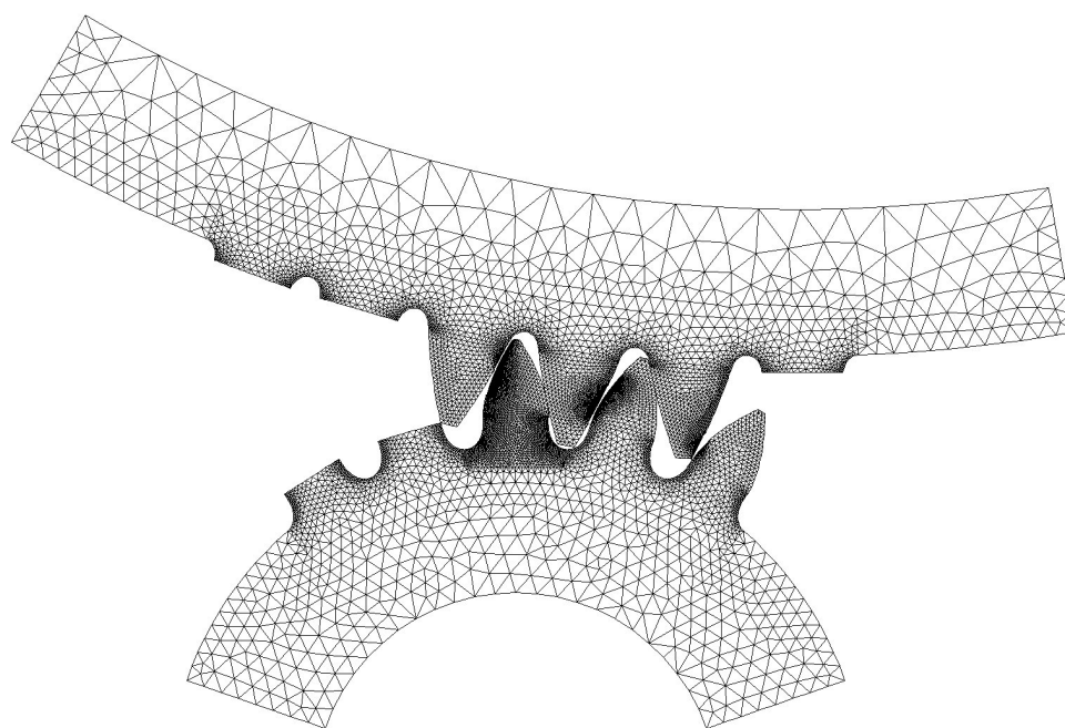
Slika 7.15 Omreženi model para zupčanika u zahvatu
