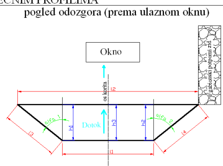
Slika 2.20. Izrada plexiglas barijere za hvatanje sitnozrnatog suspendiranog materijala
