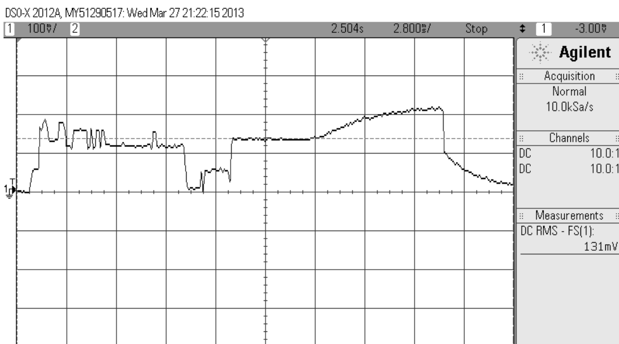
Slika 127. Mjerenja RMS napona (isprekidana linija) na otporniku od 22 Ω
