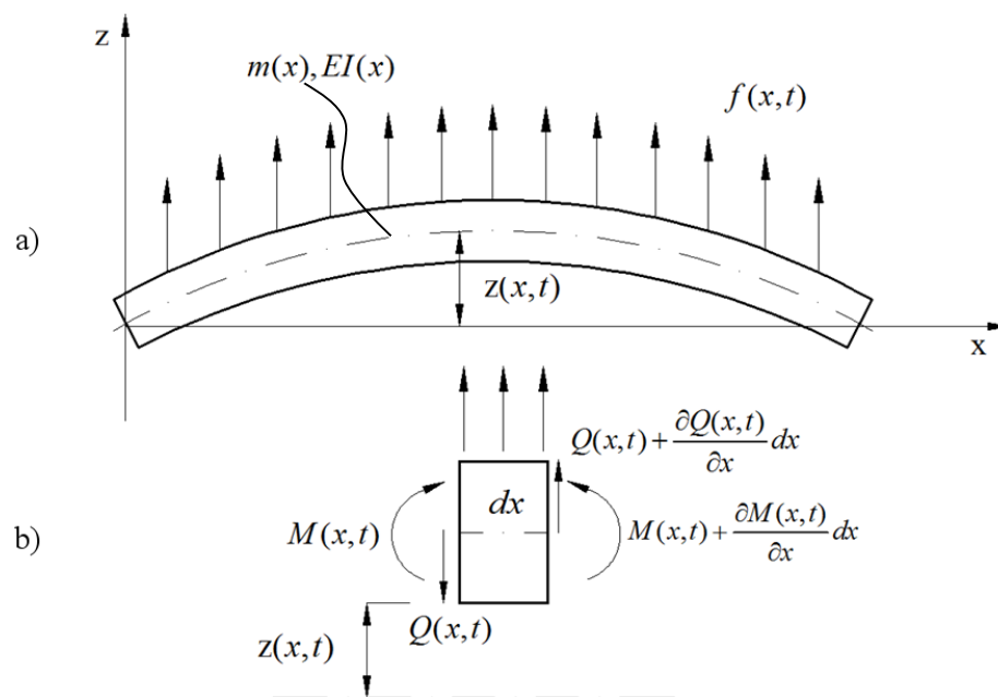
Slika 26. a) Greda pri vibracijskom savijanju i b) izdvojeni infinetezimalni segment grede diskretne širine dx s momentima i poprečnim silama [Meirovitch, 2001.]
