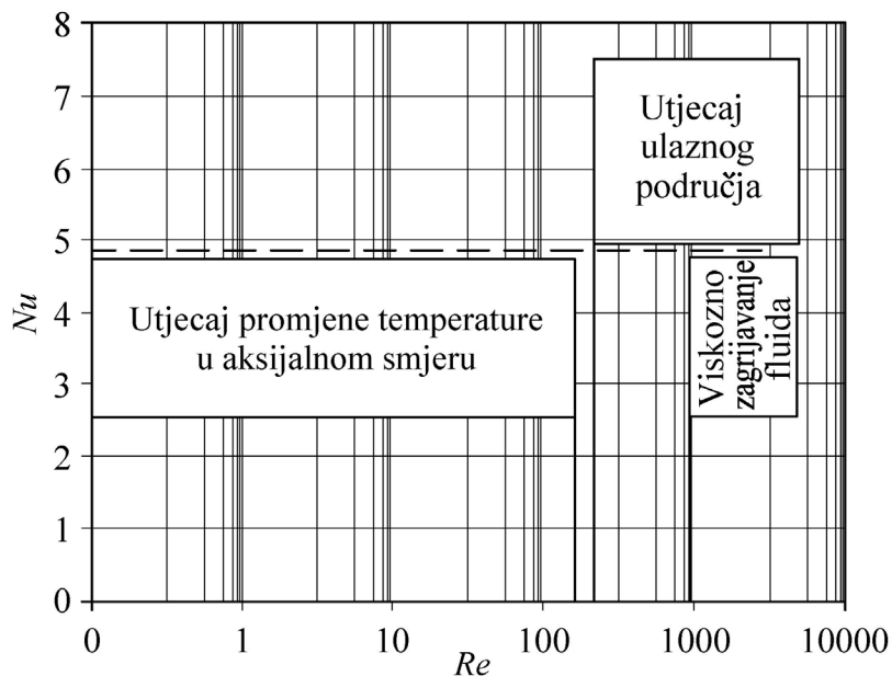
Sl. 2.14. Preporuka prema [25] za primjenu utjecaja promjene temperature u aksijalnom smjeru, utjecaja ulaznog područja i utjecaja viskozno zagrijavanja fluida na prijelaz topline u malim kanalima
