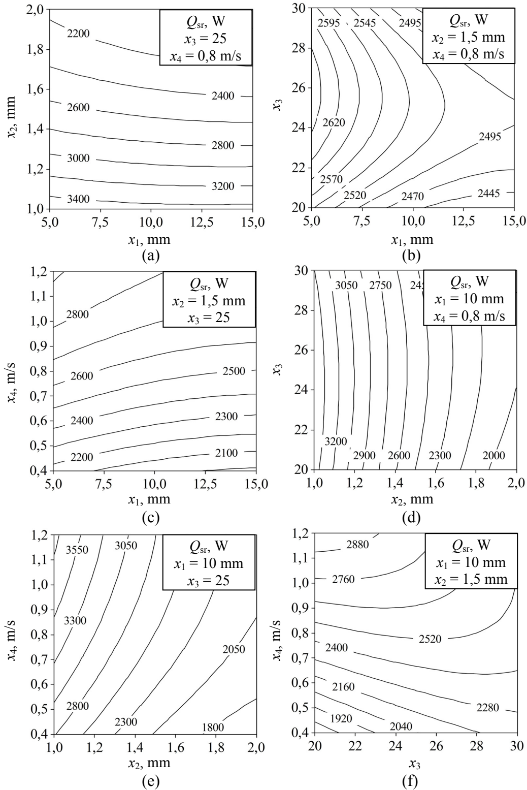
Sl. 6.9. Crteži obrisa odzivnih ploha za srednji izmijenjeni toplinski tok ( z -os, Q_{sr} ) u ovisnosti o koraku cijevi ( x_1 ), koraku lamela ( x_2 ), broju malih kanala ( x_3 ) i brzini vode na ulazu ( x_4 )
