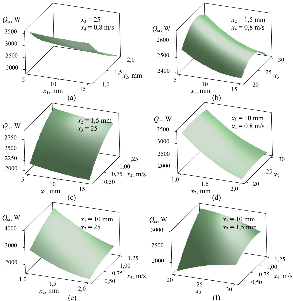
Sl. 6.7. Vizualizacija odzivnih ploha za srednji izmijenjeni toplinski tok ( z -os, Q_{sr} ) u ovisnosti o koraku cijevi ( x_1 ), koraku lamela ( x_2 ), broju malih kanala ( x_3 ) i brzini vode na ulazu ( x_4 )
