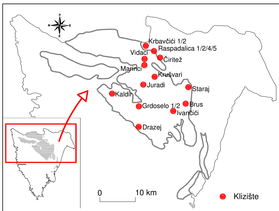
Slika 4.2 Recentna dokumentirana klizišta na flišnim kosinama središnje Istre (Dugonjič Jovančević i Arbanas 2012)
