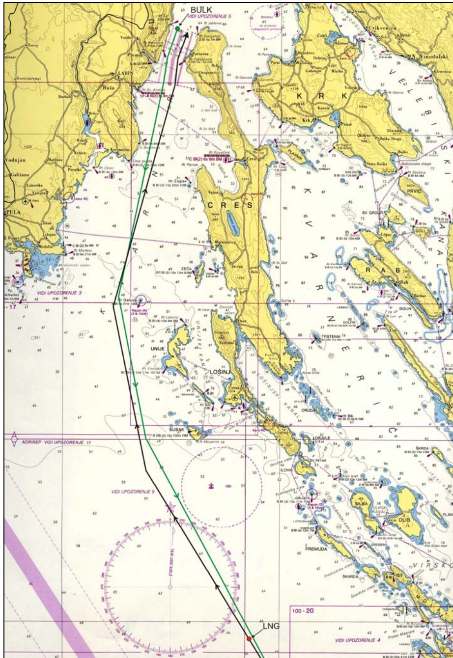
Slika 22: Segmenti plana putovanja LNG broda, broda za prijevoz rasutih tereta, te granice plovnog područja
