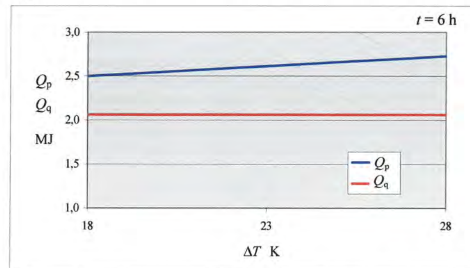
Slika 78. Utjecaj temperaturne razlike na ukupnu spremljenu toplinu i latentnu toplinu akumulatora topline pri procesu taljenja
