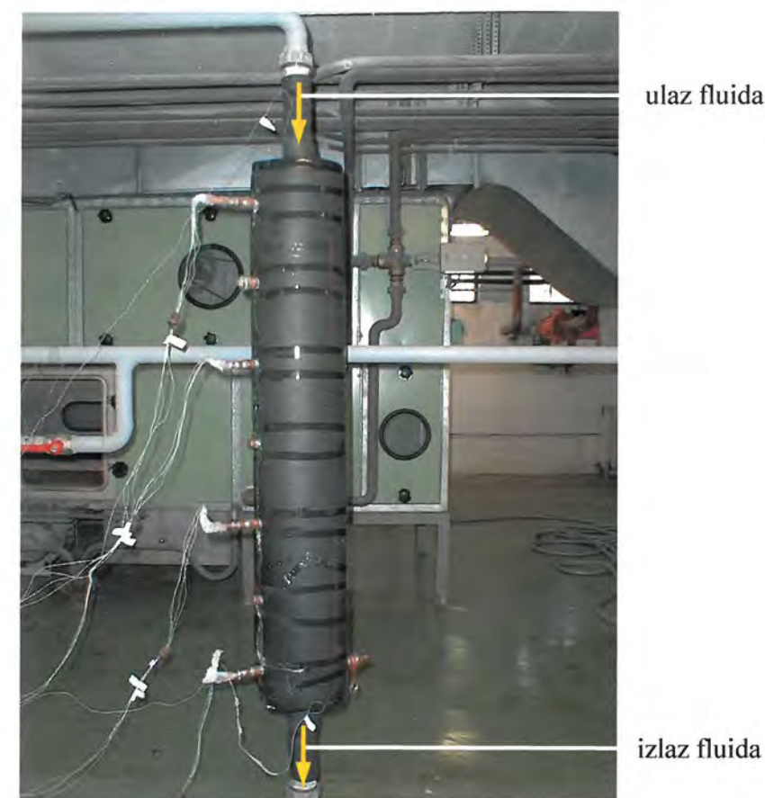
Slika 12. Eksperimentalna naprava
