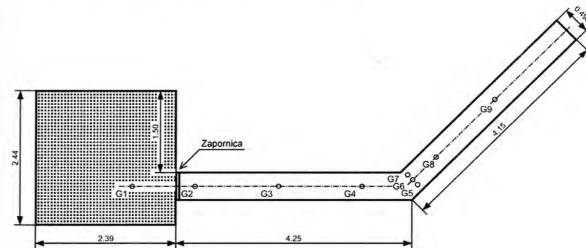
Slika 4.12. Izgled kanala s pregibom od 45^\circ
