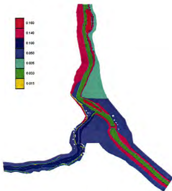
Slika 5.40. Konačno usvojene vrijednosti Manningovog koeficijenta hrapavosti
