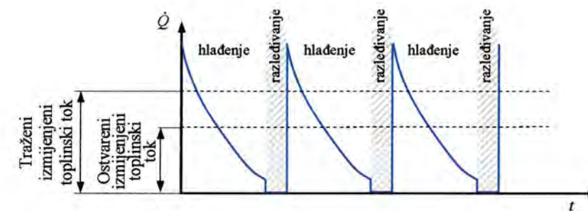
Slika 8.56. Predugačak period hlađenja u uvjetima ubrzanog nastanka ledenog sloja
