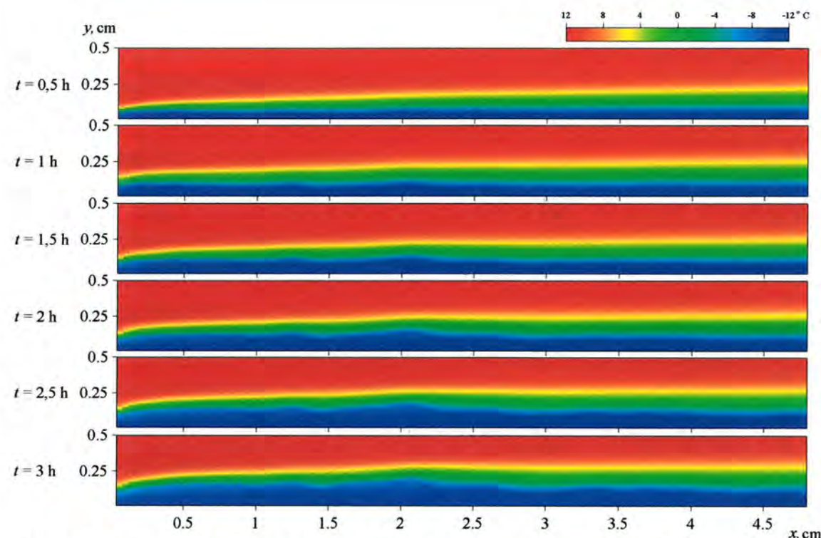
Slika 8.3. Raspodjele temperatura pri uvjetima A1 u različitim vremenima u procesu nastanka ledenog sloja
