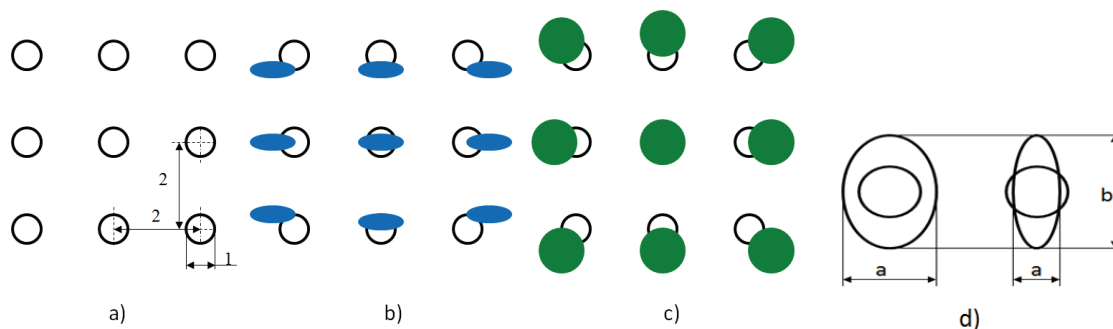
Slika 9.3 Deformacija se očituje ovisno o djelovanju napreznja, a) početni raspored kružnica (promjer 1 mm udaljenost 2 mm), b) jednoosno stanje napreznja, c) dvoosno stanje napreznja, d) shema deformiranja kružnica
