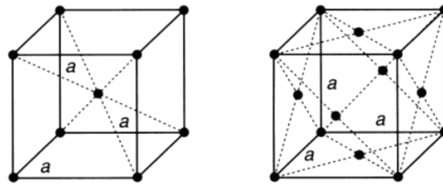
Slika 4.5 Najčešće kubične rešetke kod metala: prostorno centrirana kubična rešetka (BCC) - lijevo i plošno centrirana kubična rešetka (FCC) - desno [71, 75]
