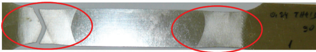
Slika 4.8 Pojava Lüdersovih traka pri izvedbi vlačnog testa, lim TH415
