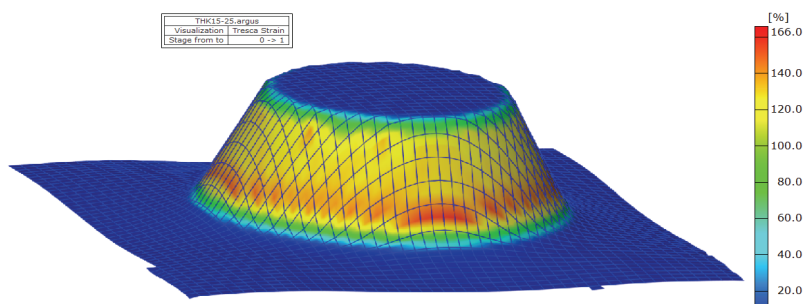
Slika 9.18 Raspodjela deformacija prema Tresca kriteriju za krnji stožac TH415 kut uzorka 63^\circ te visina 25 mm
