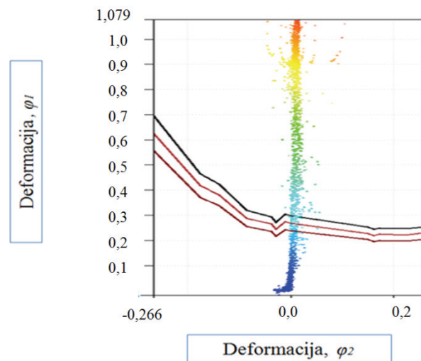
Slika 9.13 Dijagram sposobnosti oblikovanja za materijal TS230, kut od 58^\circ , visina 25 mm
