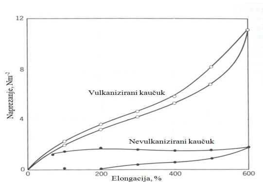
Slika 5. Ovisnost napreznja o istezanju (deformaciji) za nevulkanizirani i vulkanizirani kaučuk
