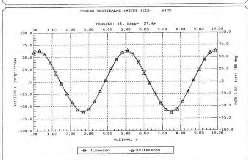
Sl. 6.13 Simulacija linearnog i nelinearnog procesa vertikalne poprečne sile (VBF) na presjeku 15 ( 3/4L_{pp} ) tri omjera valne duljine i duljine broda između okomica \lambda/L_{pp}(2,0; 1,2; 0,6) i nagib vala \lambda/a_w=80
