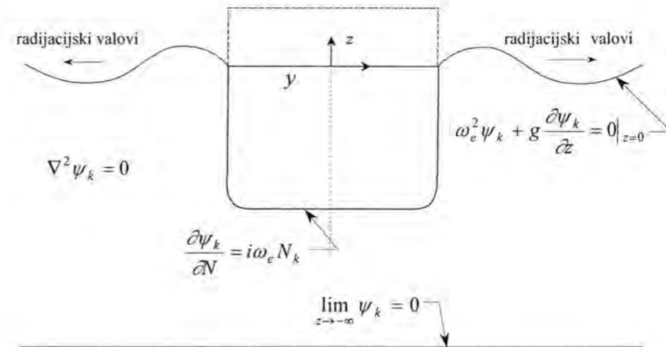
Sl. P1.1 Dvodimenzijski problem za potencijal \psi_k
