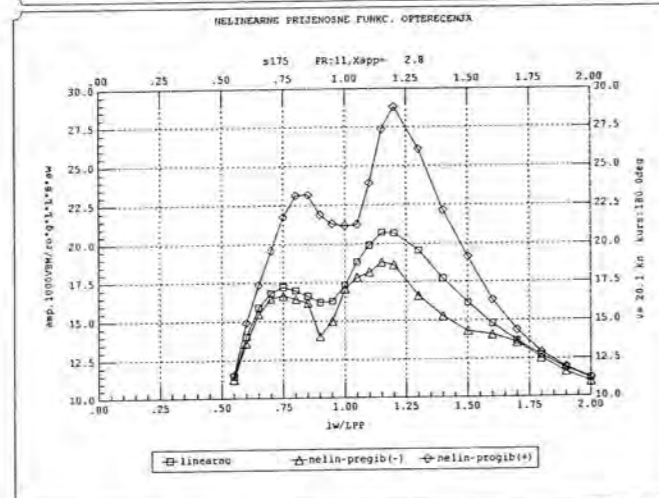
Sl. 6.16 Usporedba linearne i nelinearne prijenosne funkcije amplitude a) vertikalne poprečne sile (V3) na presjeku 15 ( 3/4L_{pp} ), b) vertikalnog momenta savijanja (VBM) na glavnom rebu (presjek 11)
