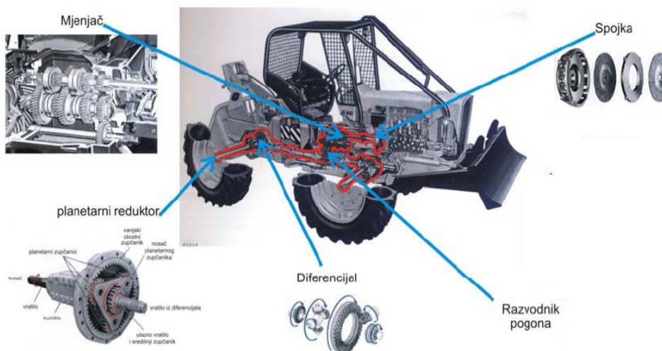
Slika 2.7. Sustav mehaničke transmisije skidera [1]
