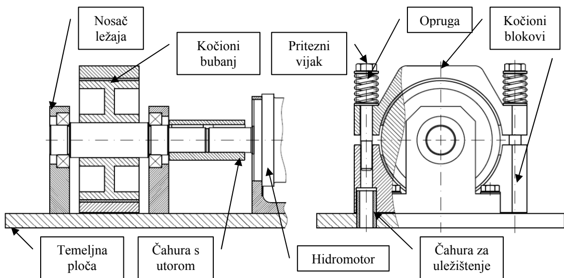
Slika 5.6. Konstruktivna izvedba veze tarne kočnice i hidromotora
